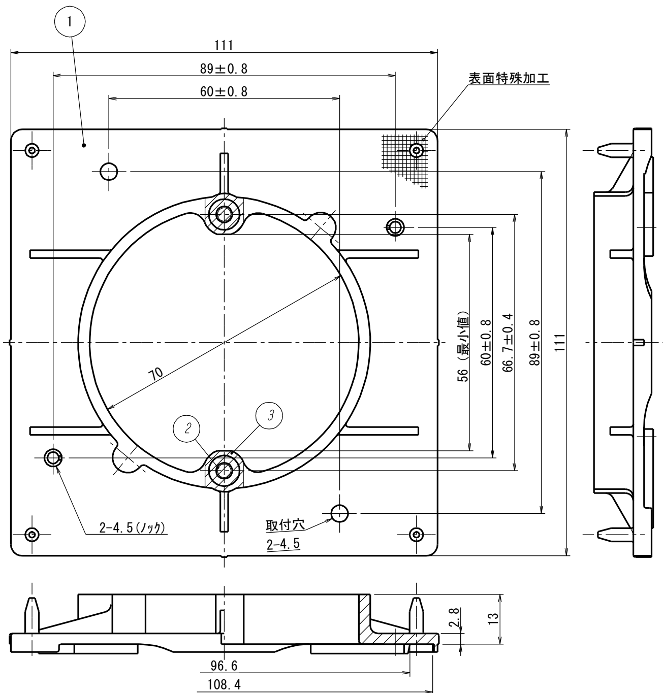
製品仕様図
